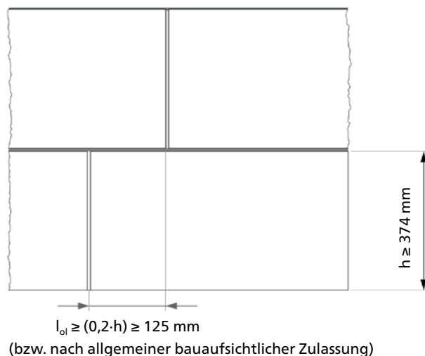
Elementmauerwerk
