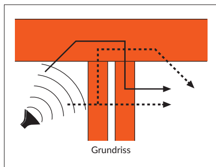
Bild 4.6: Schallübertragung bei zweischaligen Wänden aus biegesteifen Schalen mit starrem Randanschluss.
