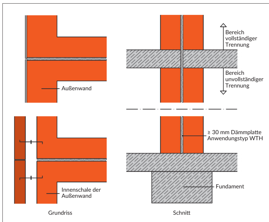
Bild 4.7: Beispiel für eine zweischalige Wand aus zwei schweren, biegesteifen Schalen mit bis zur Sohle durchgehender Trennfuge (schematisch).
