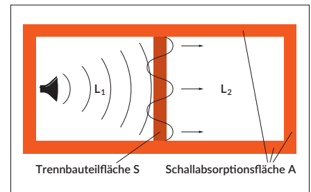
Bild 2.5: Luftschalldämmung eines Trennbauteils.
