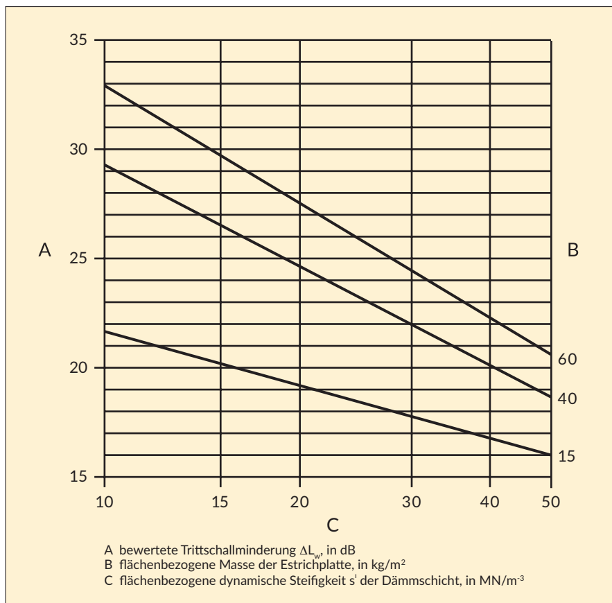
Bild 5.7: Bewertete Trittschallminderung \Delta L_w schwimmender Gussasphalt- oder Fertigteilestriche.
