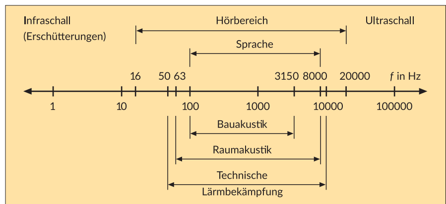
Bild 2.2: Akustischer Frequenzbereich.
